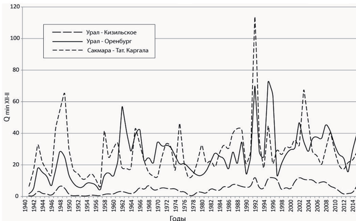
Рисунок 1 – Многолетняя динамика значений минимального среднемесячного зимнего стока рек бассейна р.Урал.
